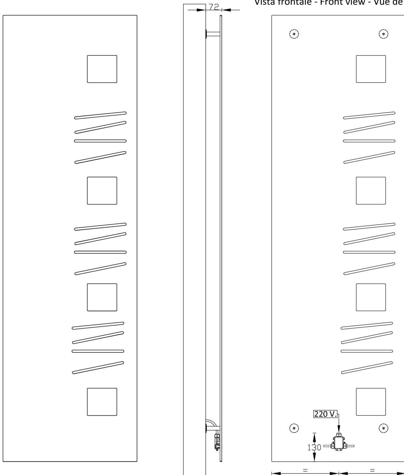
Vista frontale - Front view - Vue de face
